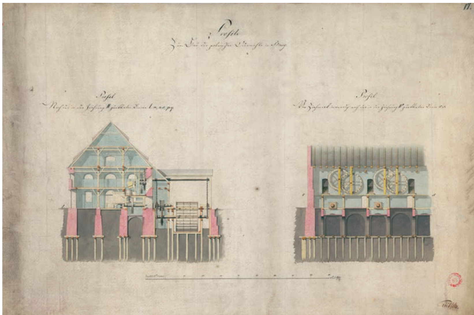
30. Brzeg. Przekrój młyna polskiego z palowaniem, 1801 Brzeg. The cross-section of the Polish mill with piling, 1801
