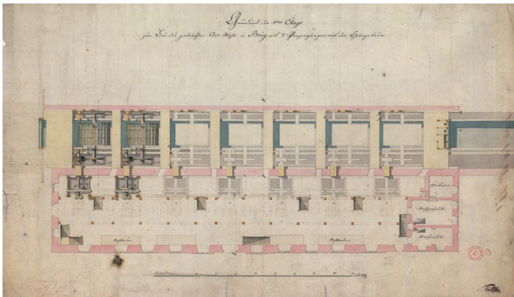
29. Brzeg. Rzut młyna polskiego z kołami napędowymi, 1801 Brzeg. The plan of the Polish mill with spinning wheels, 1801
